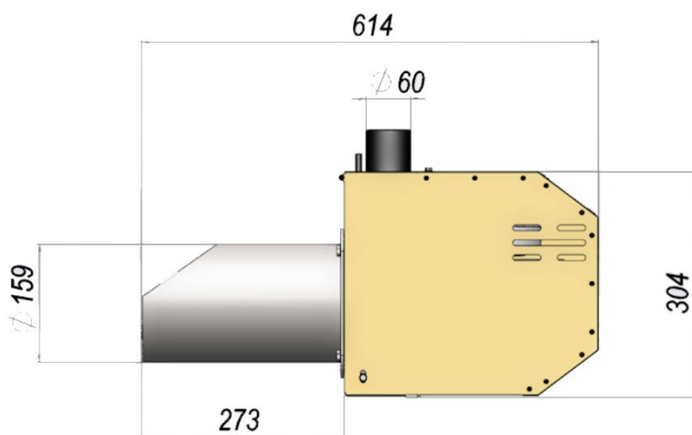
Мал. 2 – Габаритні розміри пальника «BEETERM 30»
