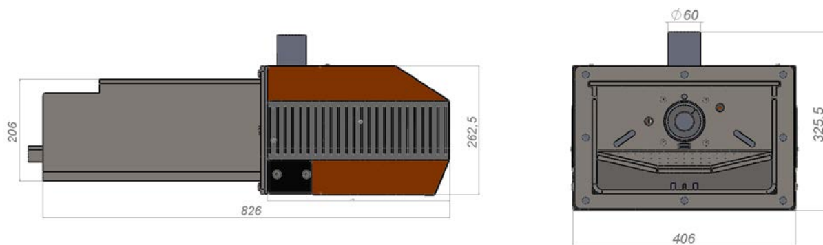
Мал. 7 – Габаритні розміри пальника «BEETERM 200»
