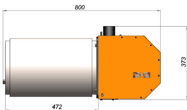
Мал. 6 – Габаритні розміри пальника «BEETERM 150»
