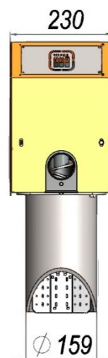
Мал. 2 – Габаритні розміри пальника «BEETERM 30»
