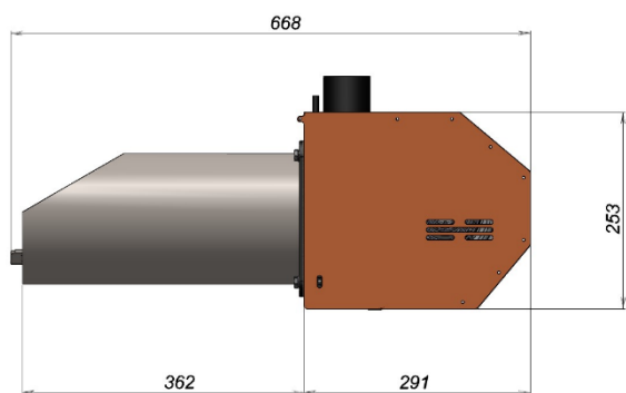
Мал. 4 – Габаритні розміри пальника BEETERM 75»
