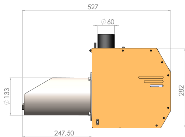
Мал. 1 – Габаритні розміри пальника «BEETERM 20»
