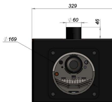
Мал. 4 – Габаритні розміри пальника BEETERM 75»
