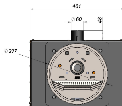
Мал. 6 – Габаритні розміри пальника «BEETERM 150»
