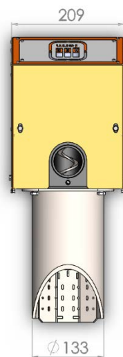
Мал. 1 – Габаритні розміри пальника «BEETERM 20»
