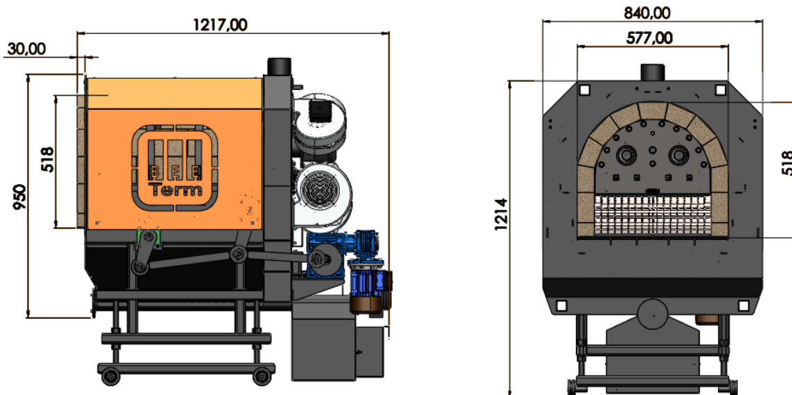
Мал. 10 – Габаритні розміри пальника «BEETERM 500»
