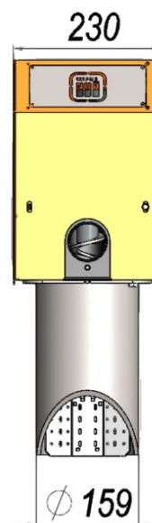
Мал. 3 – Габаритні розміри пальника BEETERM50»
