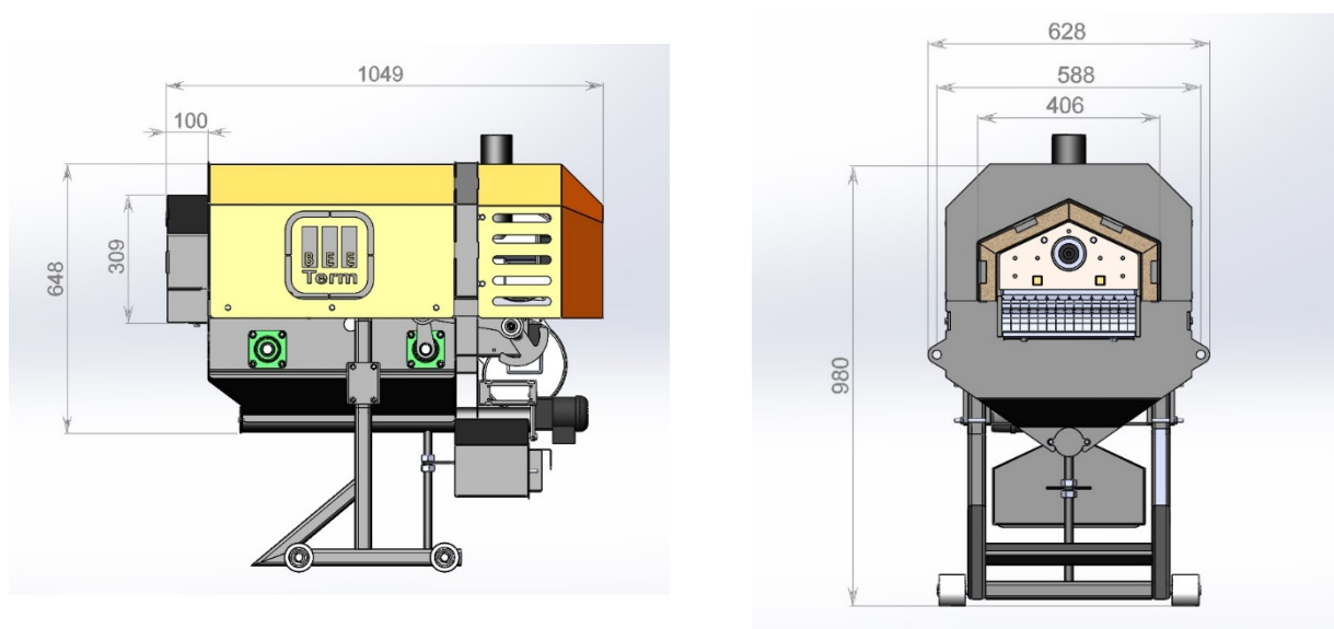
Мал. 8 – Габаритні розміри пальника «BEETERM 300»
